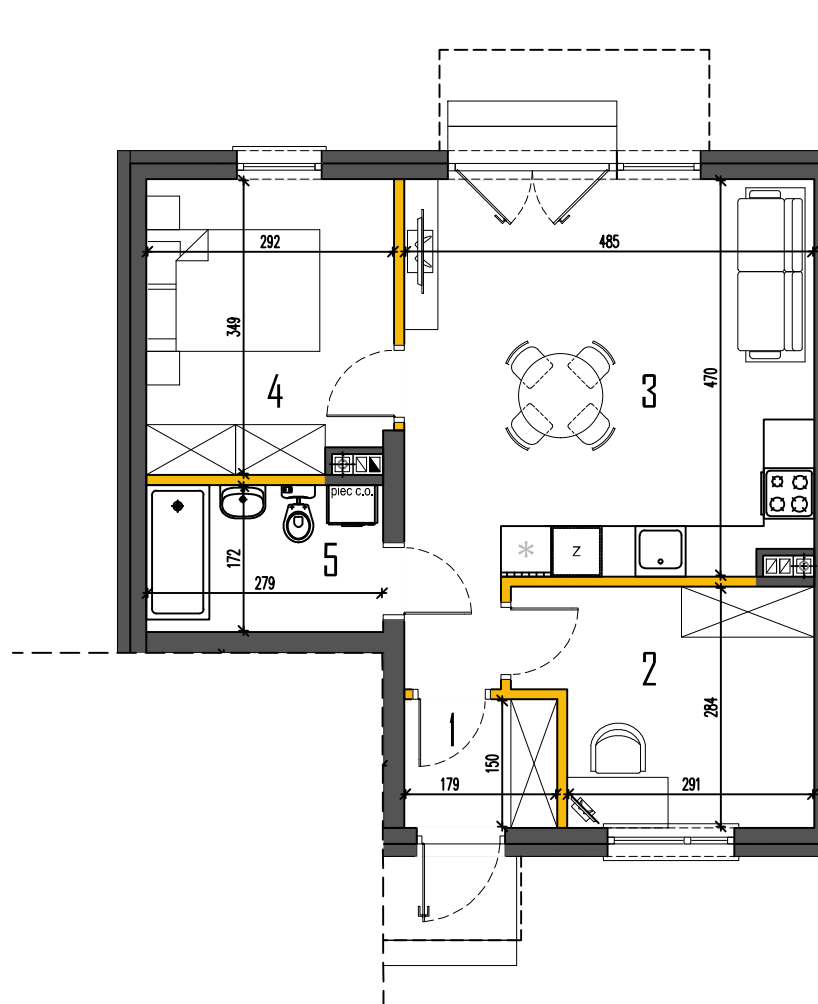
RZUT PARTERU
