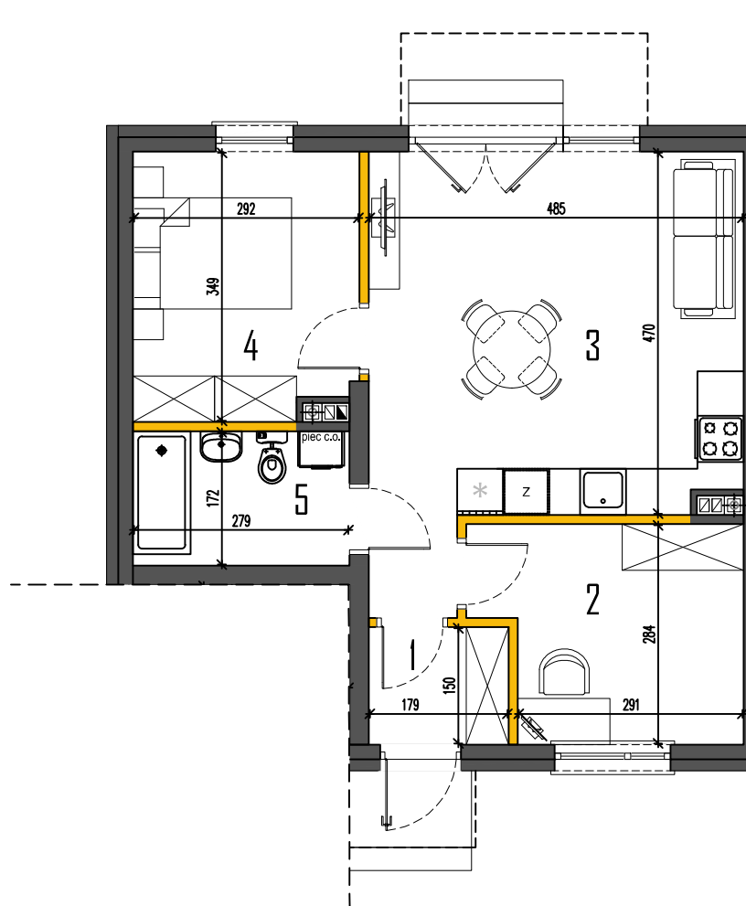
RZUT PARTERU
