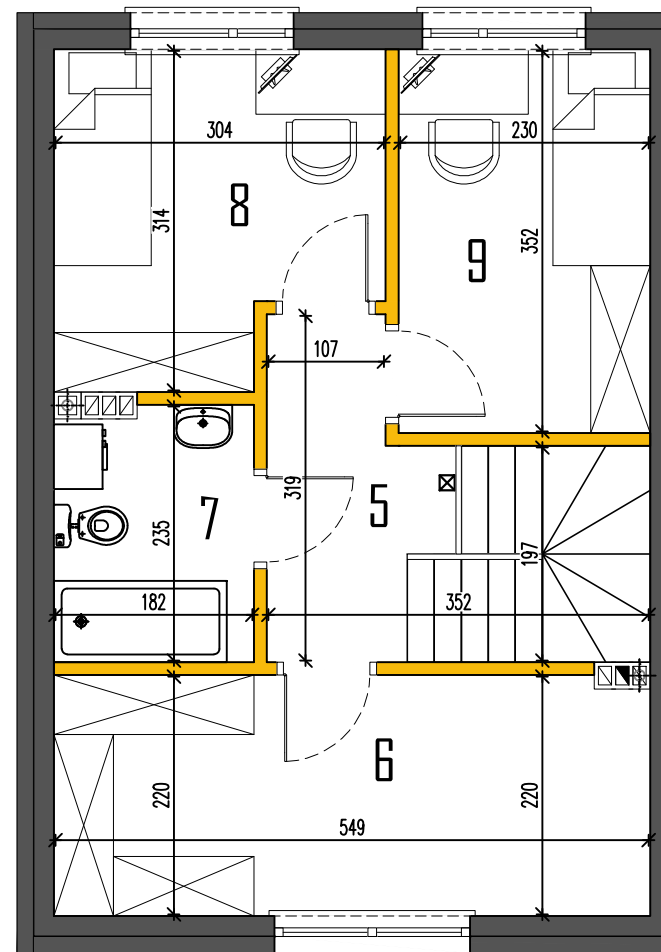
RZUT PIĘTRA
